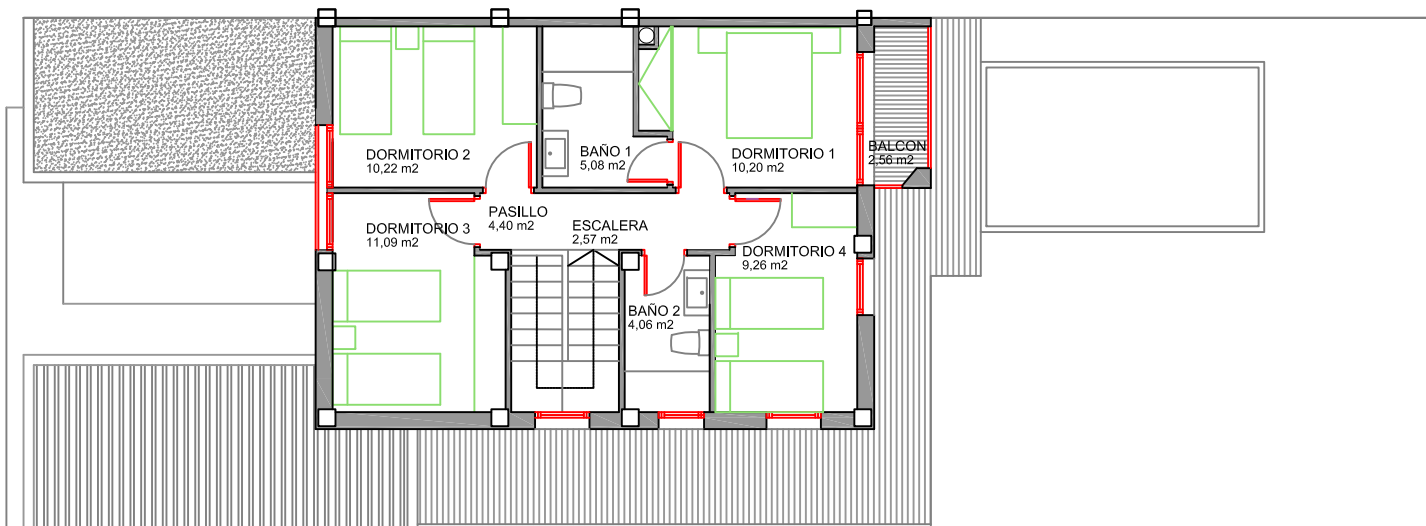
PLANTA PRIMERA
