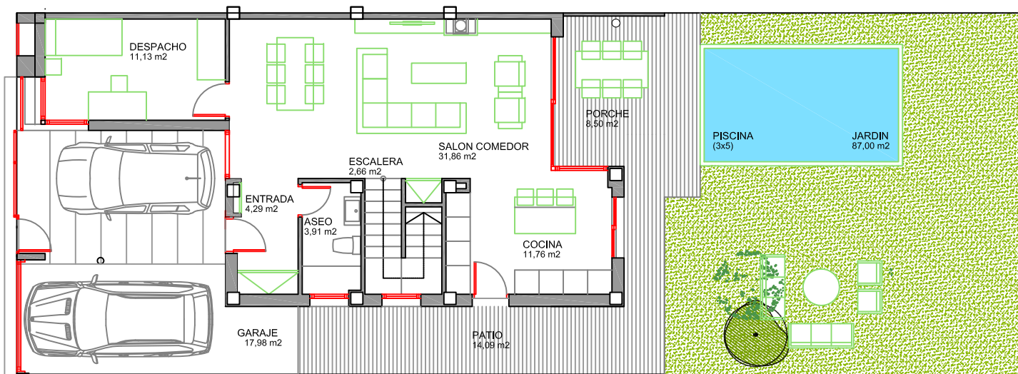
PLANTA BAJA
