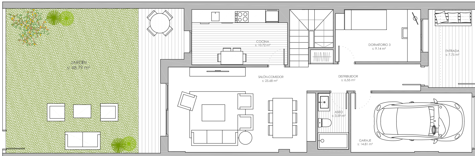
PLANTA BAJA
